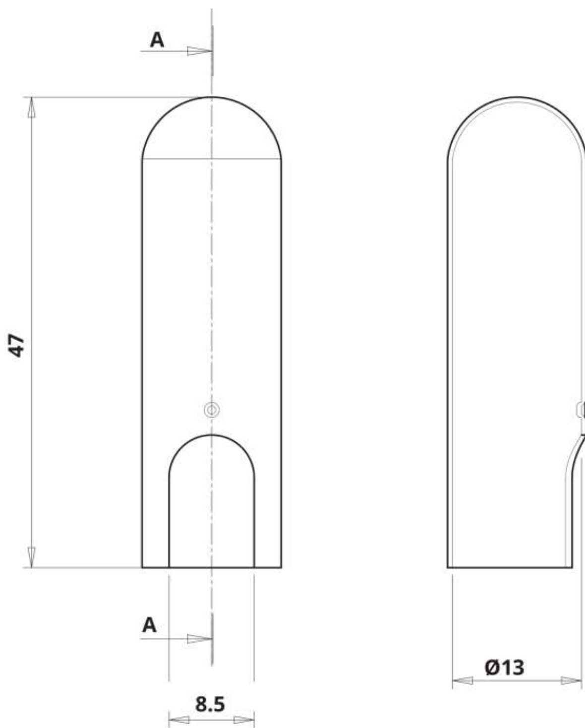
Sez. A-A
